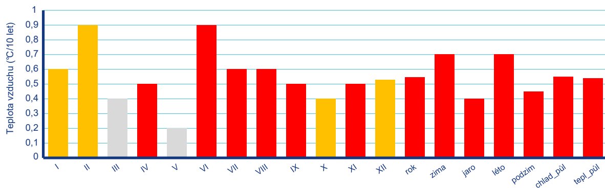
Lineární trend změny průměrné teploty vzduchu za 10 let na stanici Klementinum pro měsíce, rok a sezony v období 1981–2025. Červeně probarvené sloupčky přísluší teplotním vzestupům statisticky významným na hladině významnosti 0,01, žlutě na hladině 0,05.
